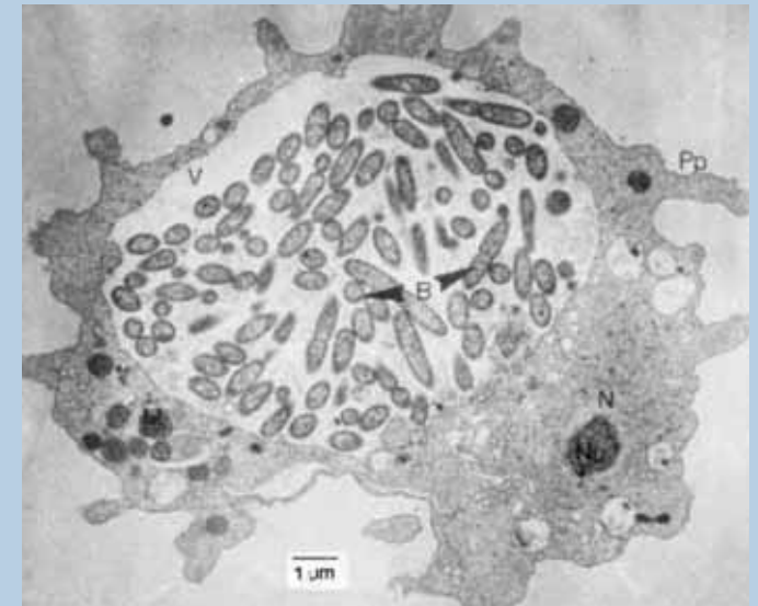
Abb. 2: Ultradünnschnitt einer Acanthamöbe mit großer, von Legionellen erfüllter Vakuole. Virulenter Phänotyp, erkennbar an den Speicherkörperchen (durch Pfeile markiert). Elektronenmikroskop, 3000x. Originalaufnahme Univ. Prof. Tiefenbrunner
