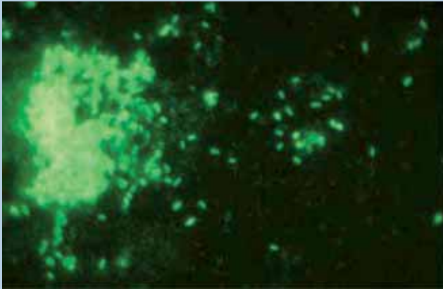
Abb. 3: Austreten der vermehrten Legionellen (FITC-Fluoreszenzantikörper markiert) aus einer zerstörten Amöbe (nicht angefärbt). Originalaufnahme Univ. Prof. Tiefenbrunner
